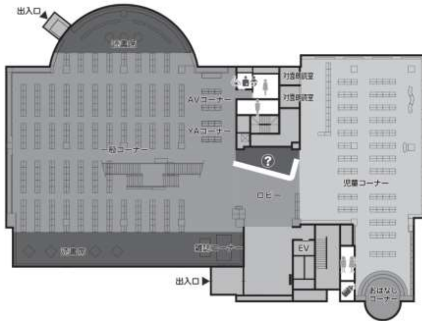
【1階平面図】
