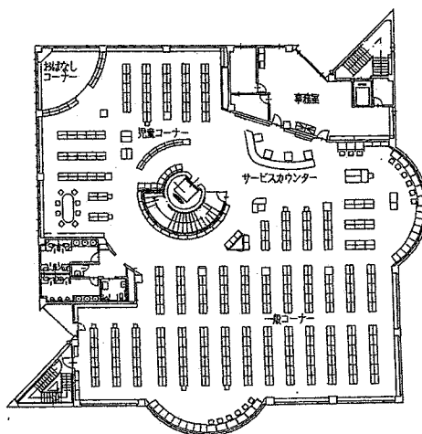
2階平面図
